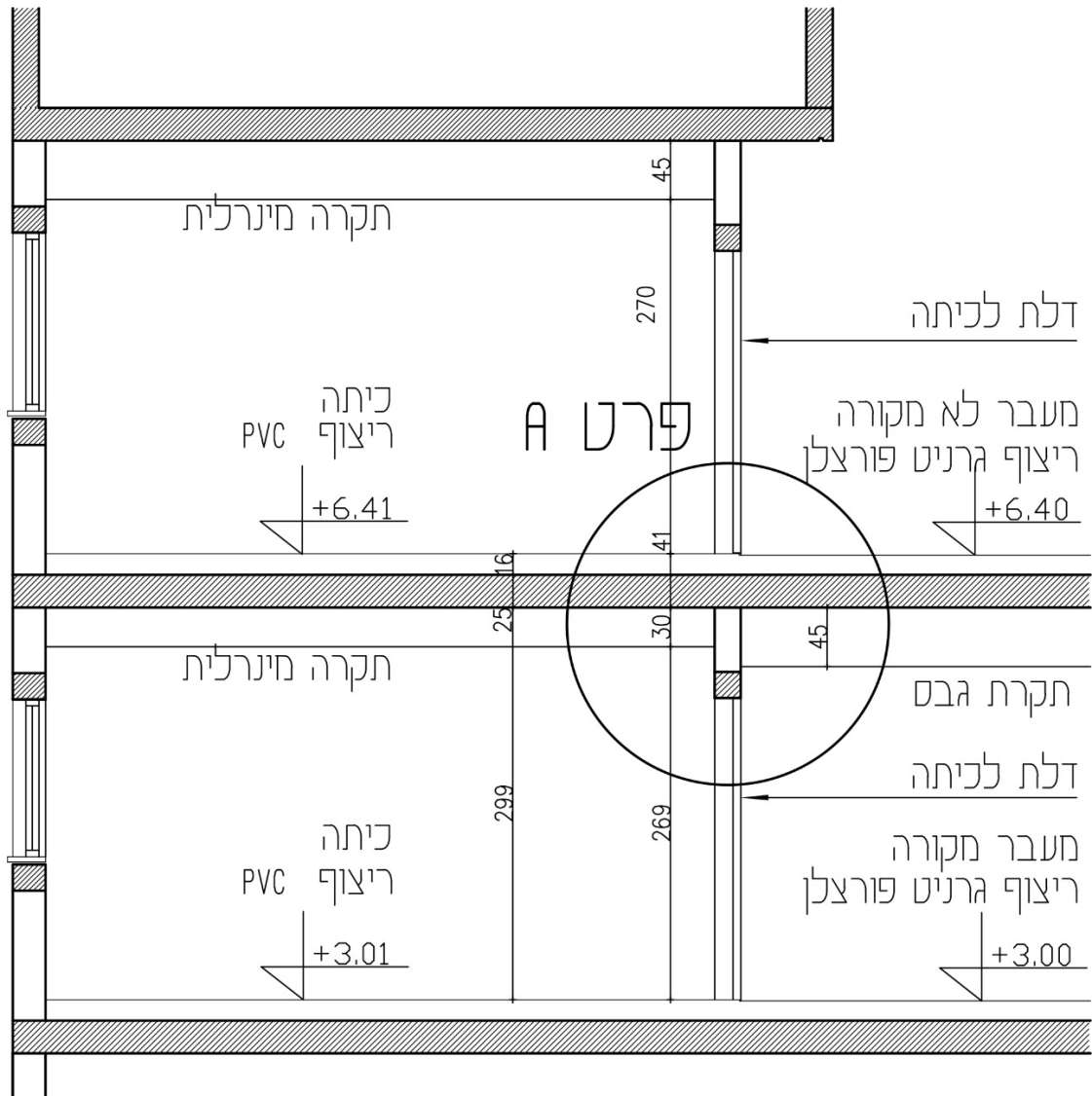
חתך דרך כיתה ומעבר
