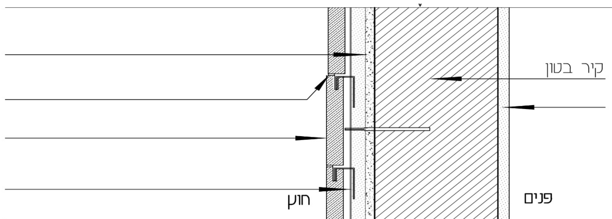
פרט 1- קיר בטון בחיפוי טיח ואבן
