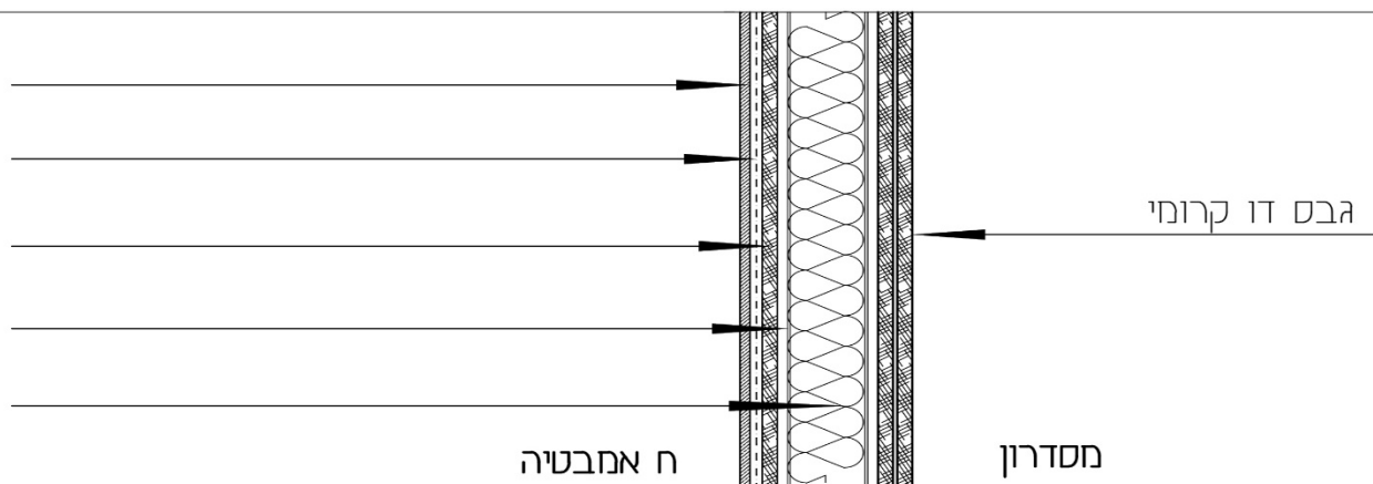
פרט 2- קיר גבס בחיפוי גרניט פורצלן
