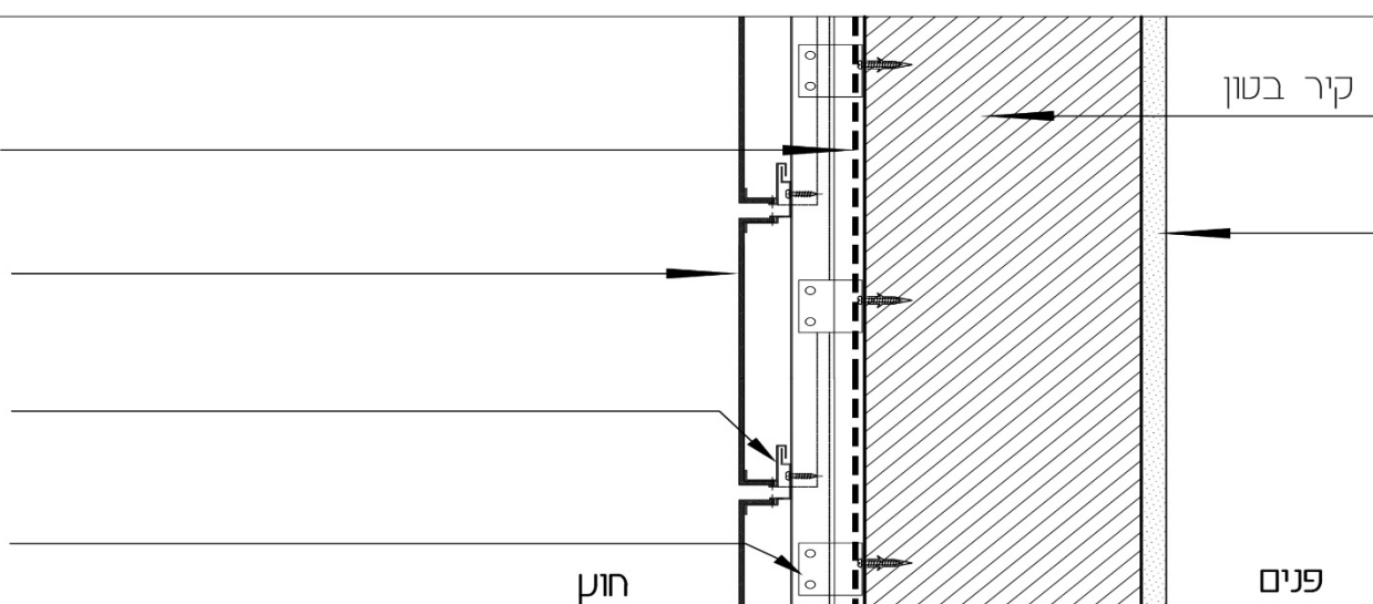
פרט 3- קיר בטון בחיפוי טיח ולוחות אלומיניום
